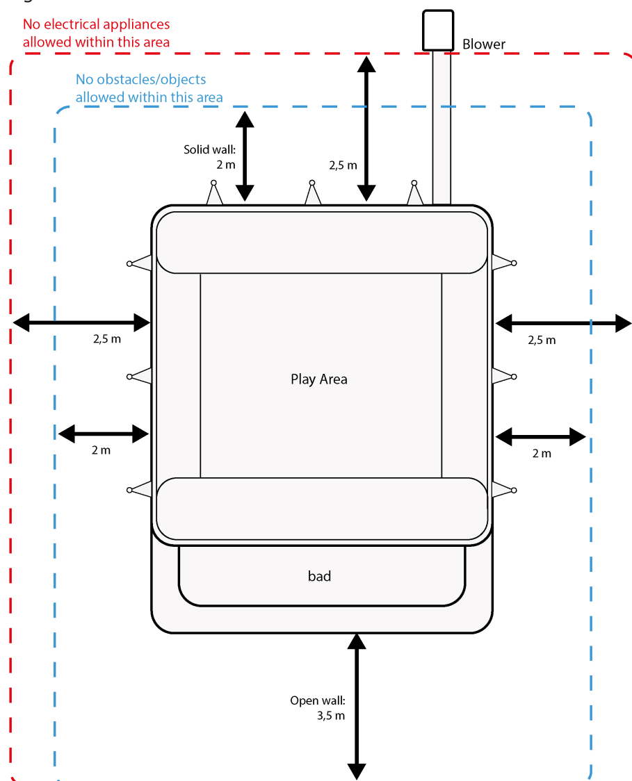
Figuur 2 Minimale vereiste vrije ruimtes rondom het springkussen.
